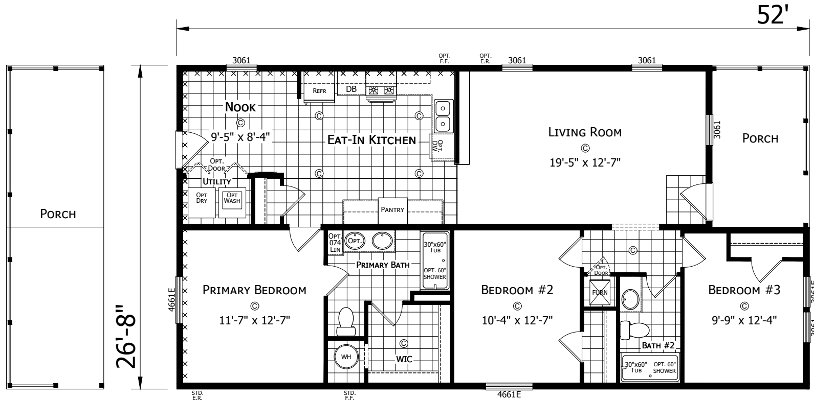
OPTIONAL PORCH
